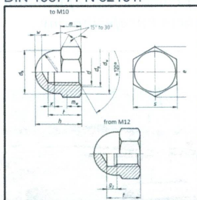
Rys 20 Nakrętka kołpakowa.
